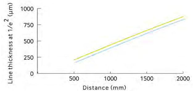
Darstellung der Fokussierungswerte Quelle: global-laser.co.uk
