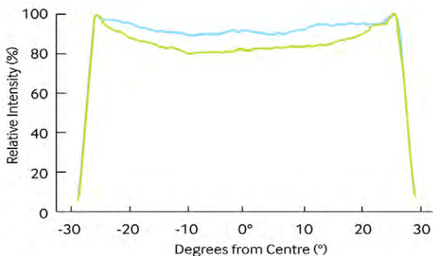
Gleichmäßige Leistungsverteilung Quelle: global-laser.co.uk
